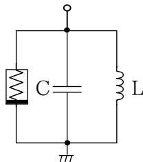
Fig. 1. van der Pol oscillator.
